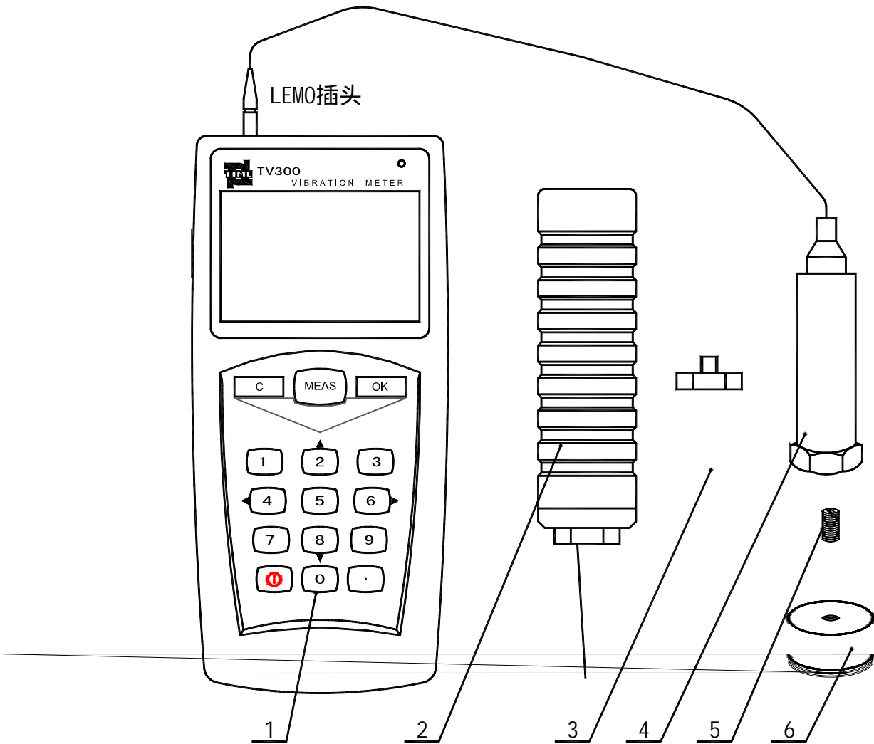
1. 主机 2. 触针组件 3. 长触针 4. 测振探头 5. 螺柱 6. 磁性吸座
